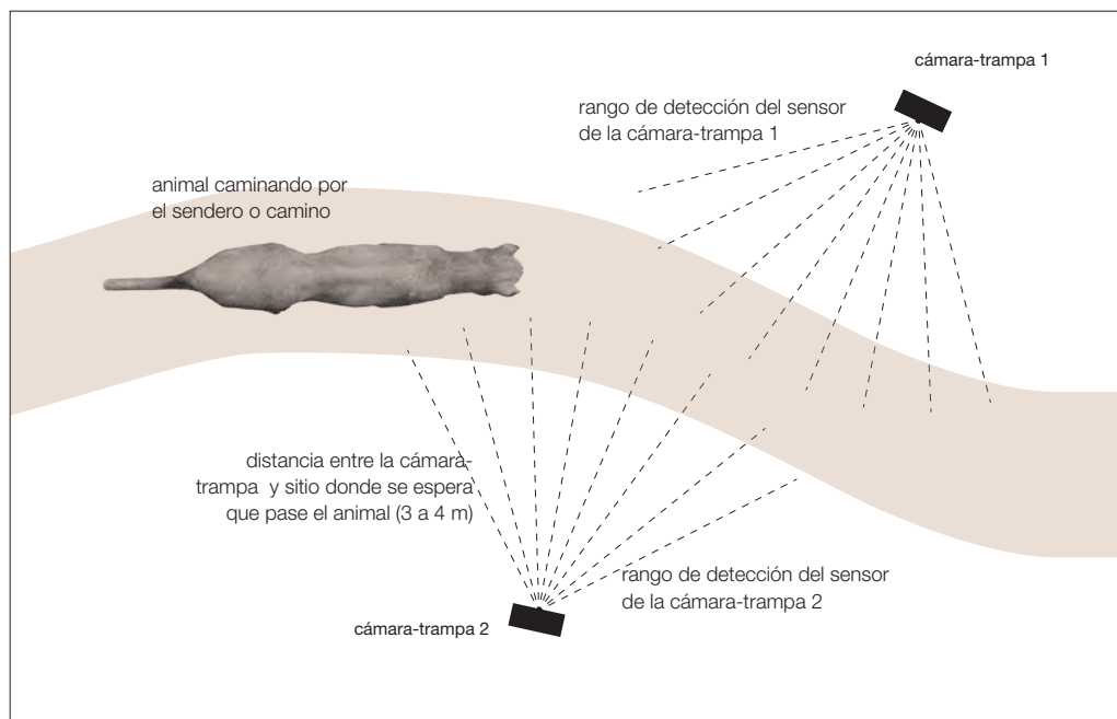
FIGURA 19. Posible distribución de las estaciones dobles (vista superior). La ilustración muestra el desfase que debe existir entre las dos trampas-cámara para evitar que el flash interfiera en las imágenes. En este caso el animal que va caminando por el sendero será detectado por el sensor de la trampa-cámara 2 y fotografiado, para posteriormente ser detectado por el sensor de la trampa-cámara 1 y ser fotografiado por esta última. Imagen: A. de la Torre.
