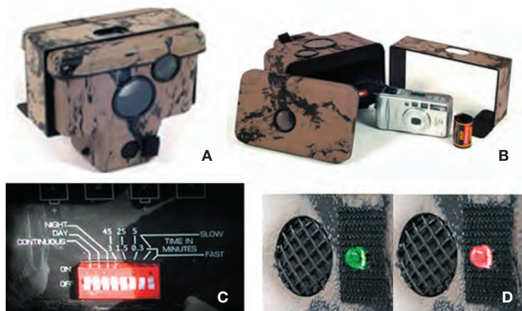
FIGURA 10. Componentes de una trampa-cámara: A) dispositivo completo; B) elementos de la trampa-cámara; C) controlador del sensor detector de movimiento y/o calor; D) forma del sensor en su modo de prueba (rojo) y en su modo de activado (verde). Fotos: <www.camtrakker.com>.
